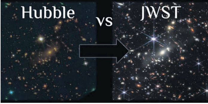
Fig.1: La première image du télescope James Webb montre des galaxies formées peu après le Big Bang, il y a plus de 13 milliards d'années.
