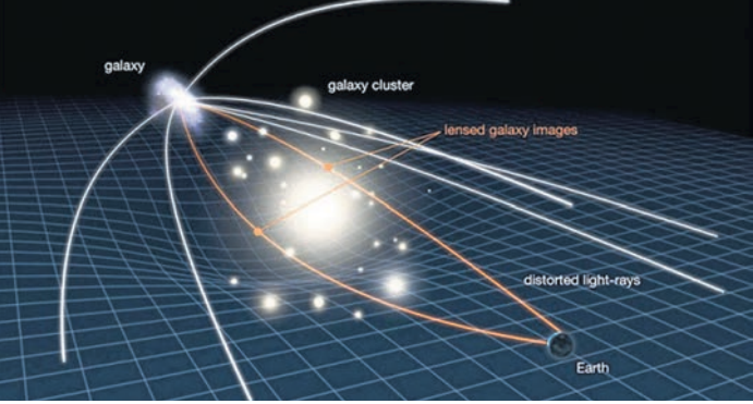
Fig.2: La déformation des images grâce à l'effet de la lentille gravitationnelle
